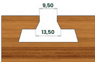
FRESA CANALETADA 18L2823.06
